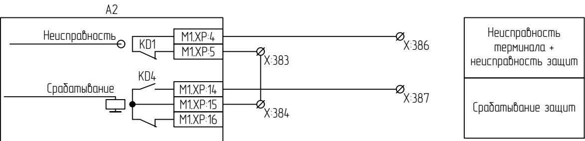
Цепи РАС
