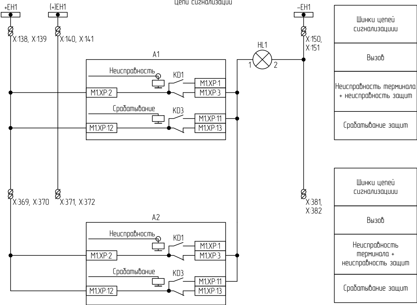
Цепи сигнализации
