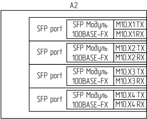
Цепи портов связи терминала
