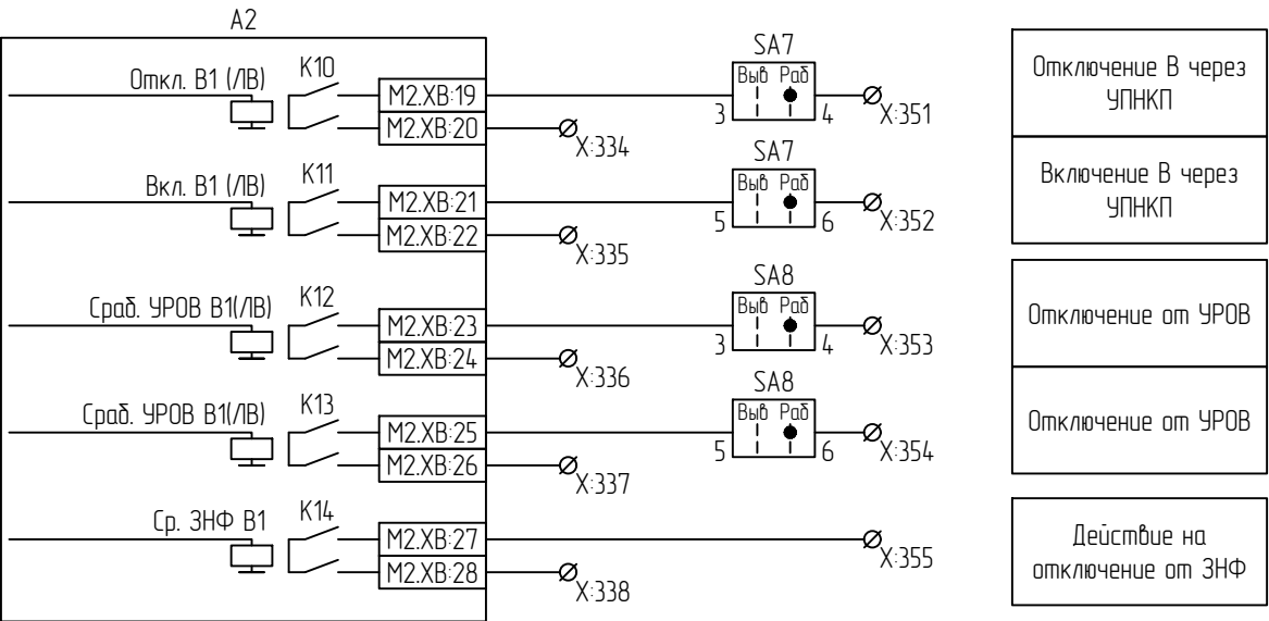
Цепи РАС
